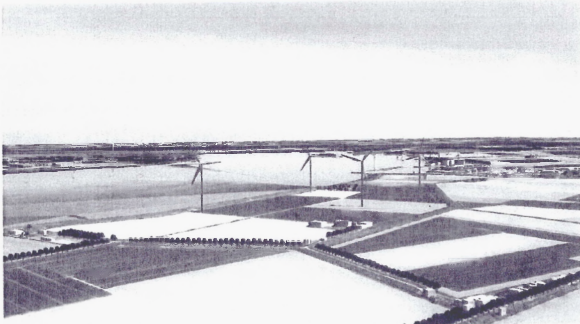
Impressie van de clusteropstelling met een rotordiameter 120 meter. Deze impressie sluit aan bij de opstellingsvariant met een tiphoogte van ongeveer 180 meter. (bron: ROM 3D)
